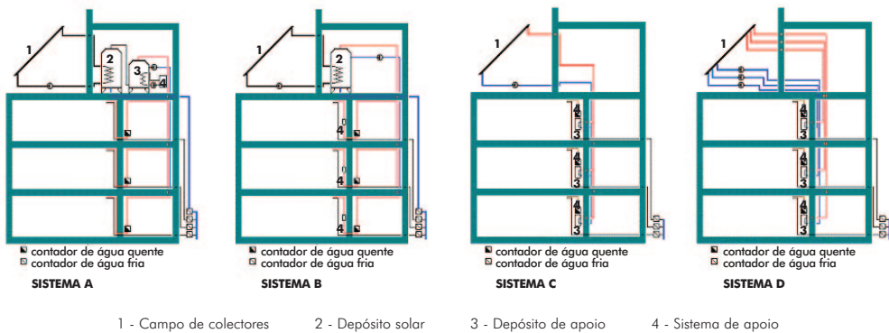
Figura 6 A, B - Sistema totalmente centralizado – Sistema centralizado com apoios individuais C, D - Campo de colectores – Sistemas individuais
